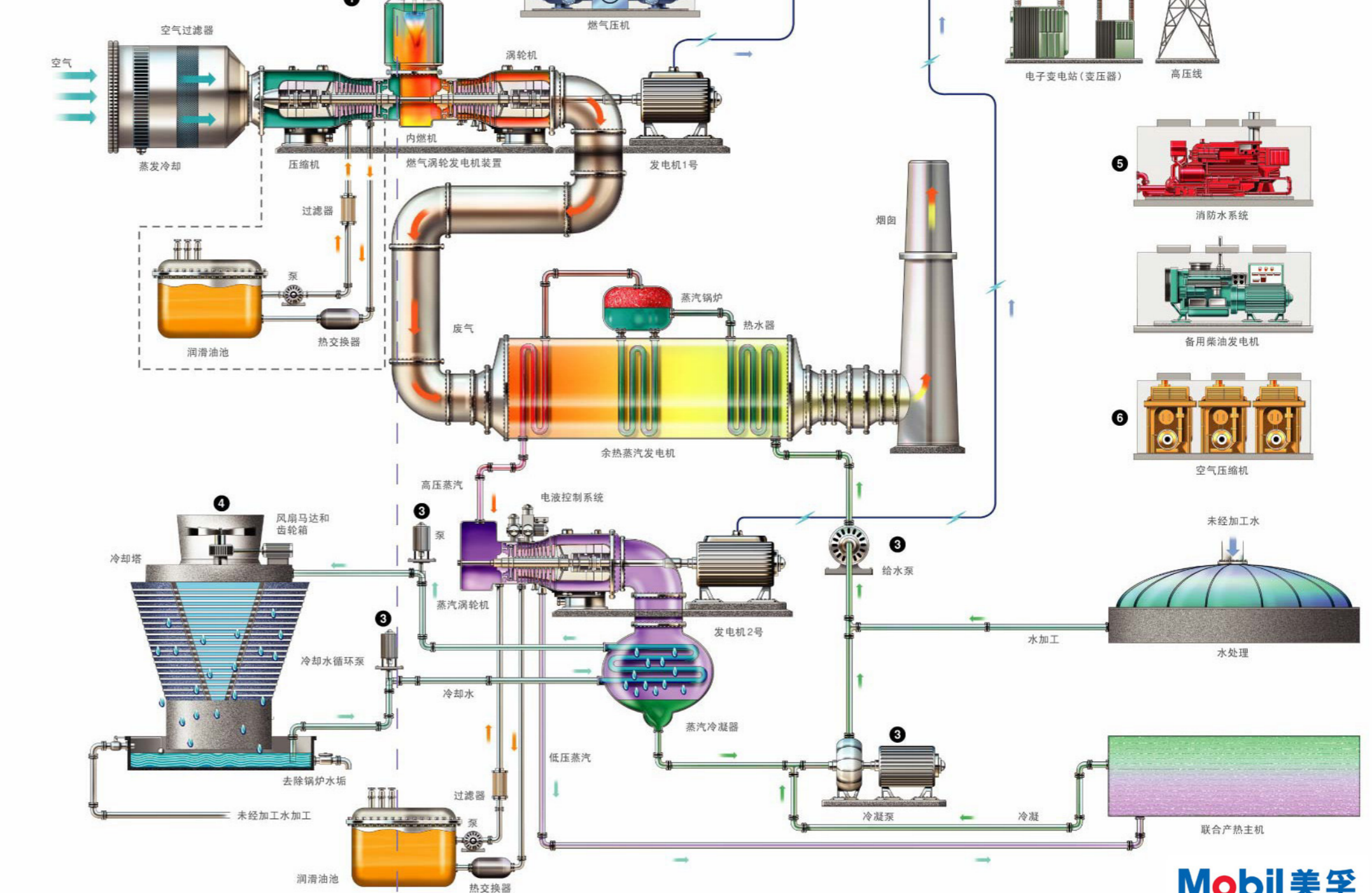
双轴燃气及蒸汽轮机发电机组
