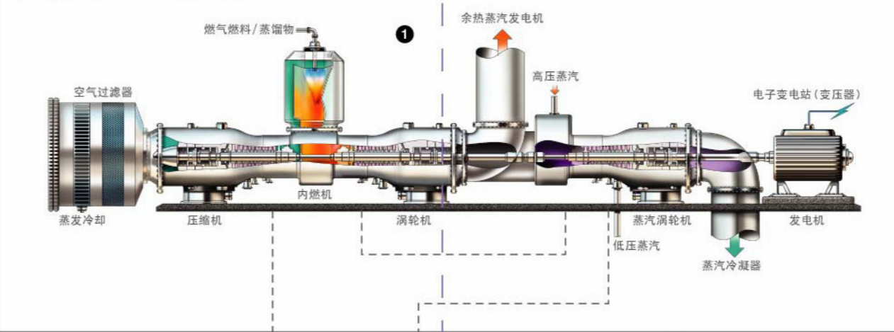
单轴燃气轮机组合循环机组
